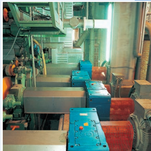
Transmisión multi-motor Multi-motor transmission set Многомоторная трансмиссия
